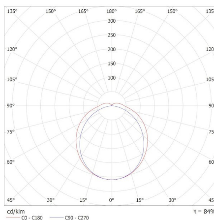
KANLUX S.A. (kat 33169) TP STRONG LED 60W-NW / Krzywa rozsyłu światła (biegunowo)
