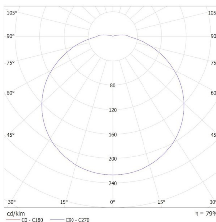
KANLUX S.A. (kat 37291) IPER LED 19W-NW-O / Krzywa rozsyłu światła (biegunowo)
